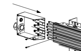
Концевой элемент питания
