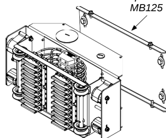
Опорный кронштейн РСТ10-MB125
