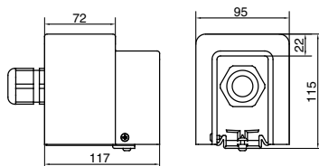
EB40 (открытый)
